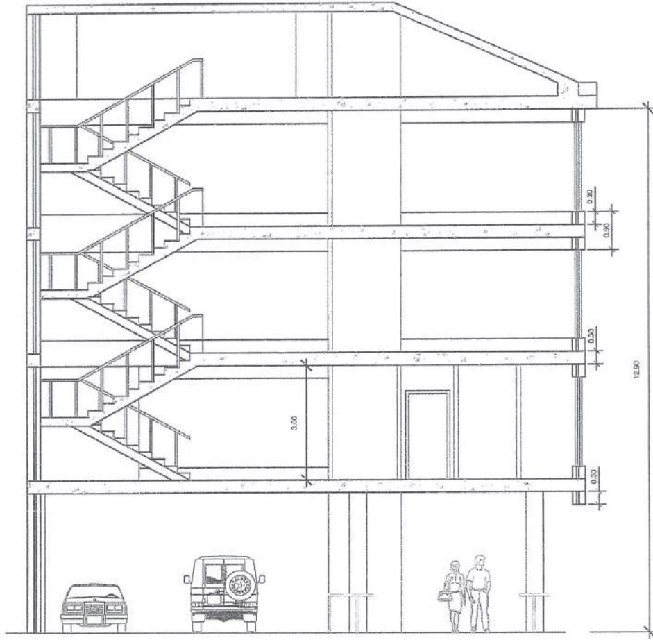
Plano 1: Edifício
